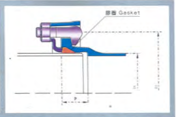
机械式快速接口 (Mechanical express joint)
